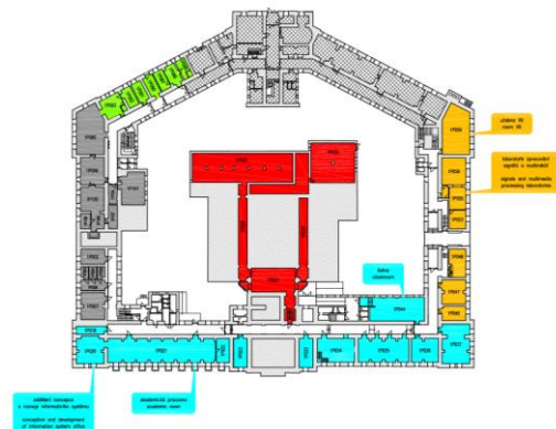
Orientační plán, 1. pozemní podlaží 1
