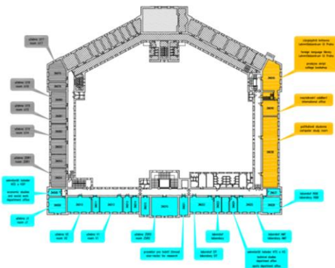
Orientační plán, 3. nadzemní podlaží 1
